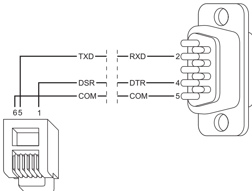
Rys. 23. Sposób podłączenia drukarki przy pomocy wtyku męskiego DB-9 (widok od strony punktów lutowniczych).
