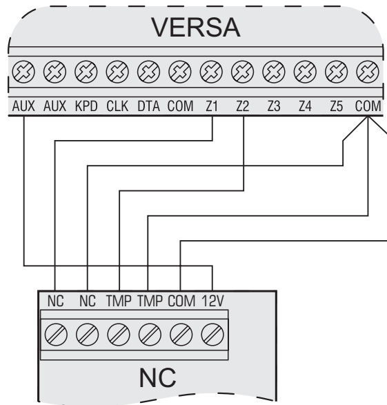
Rys. 21. Przykład podłączenia do centrali czujki typu NC (czujkę typu NO podłącza się identycznie).
