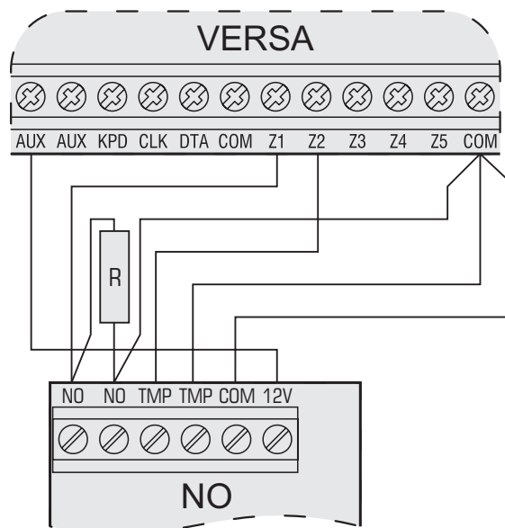
Rys. 22. Przykład podłączenia do centrali czujki typu NO w konfiguracji EOL.
